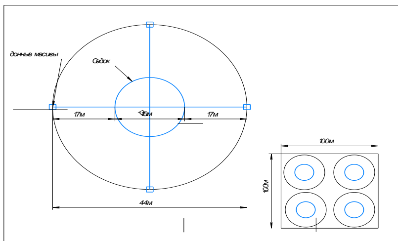
Рисунок – Схема штормоустойчивого садка для товарного выращивания белуги в условиях Азовского моря
