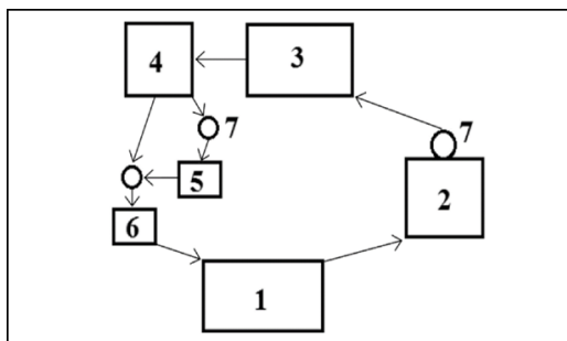
Рисунок 1 – Принципиальная схема УЗВ с блоком инкубации икры:
