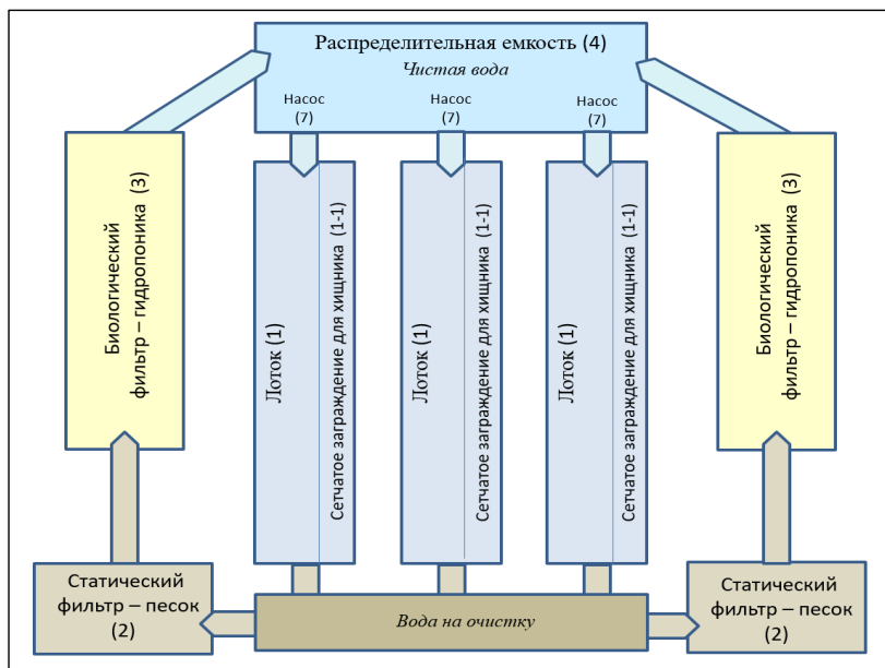
Рисунок 2 – Принципиальная схема УЗВ для тренинга рыб
